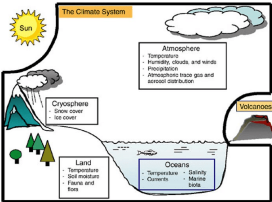
El sistema climático. Nótese que el sol, los volcanes y las actividades humanas están todos fuera del sistema climático. Fuente: NRC 2005. HT Pielke Sr.
